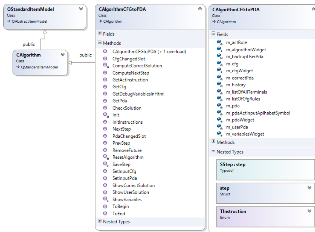
Obr. 11.3 Diagram tříd třídy CAAlgorithmCFGToPDA
