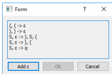
Obr. 10.5 Okno dialogu pro vkládání přechodová pravidla v zásobníkovém automatu
