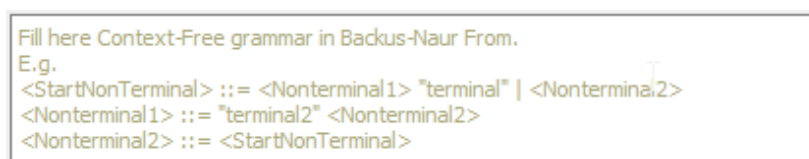
Obr. 10.2 Předvyplněný text bezkontextové gramatiky
