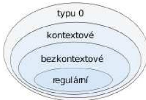
Obr. 1.1 Chomského hierarchie formálních jazyků
