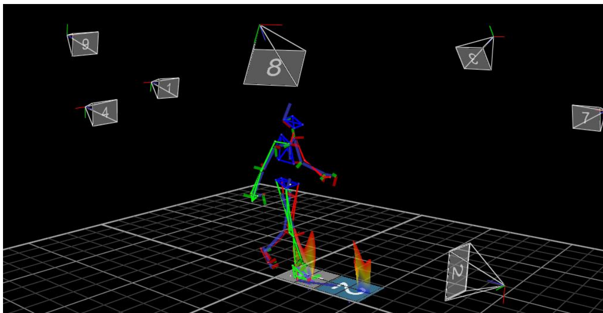
Obr. 4 Ukázka rozmístění jednotlivých kamer v Laboratoři chůze (rozmístění kopíruje uložení „ovál“)
