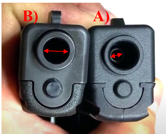
Obr. 19 Detail válcového ústí hlavně obou vzorků [vlastní]
